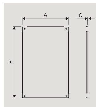
PMSL - oceľová montážna doska
