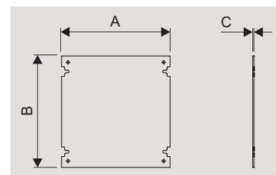
PMPL - polyesterová montážna doska
