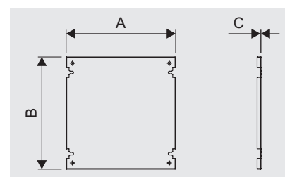
PMSL - oceľová montážna doska
